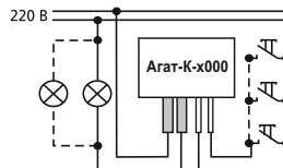
Рис.1. Схема монтажа для ламп 220 В
