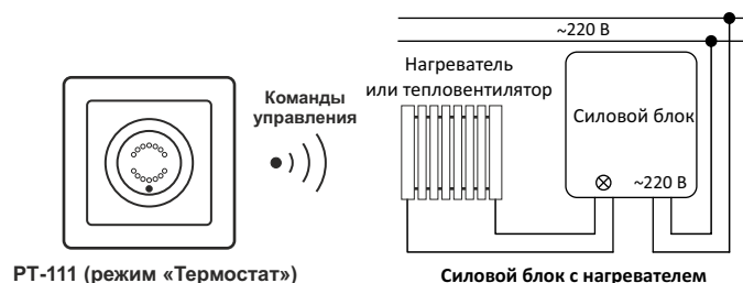
Рисунок 3. Использование датчика PT-111 в качестве термостата
