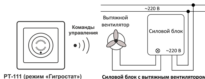
Рисунок 4. Использование датчика PT-111 в качестве гигростата
